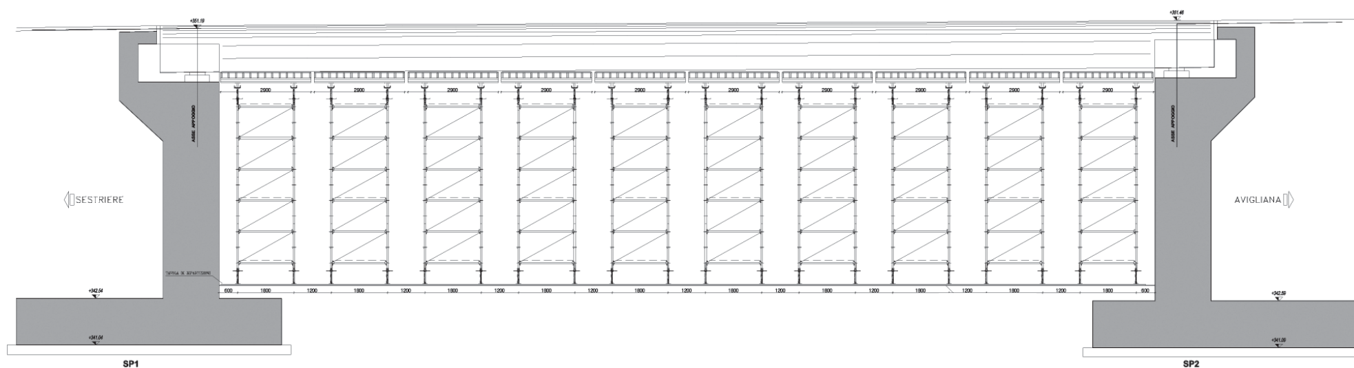
SEZIONE LONGITUDINALE - Longitudinal section
